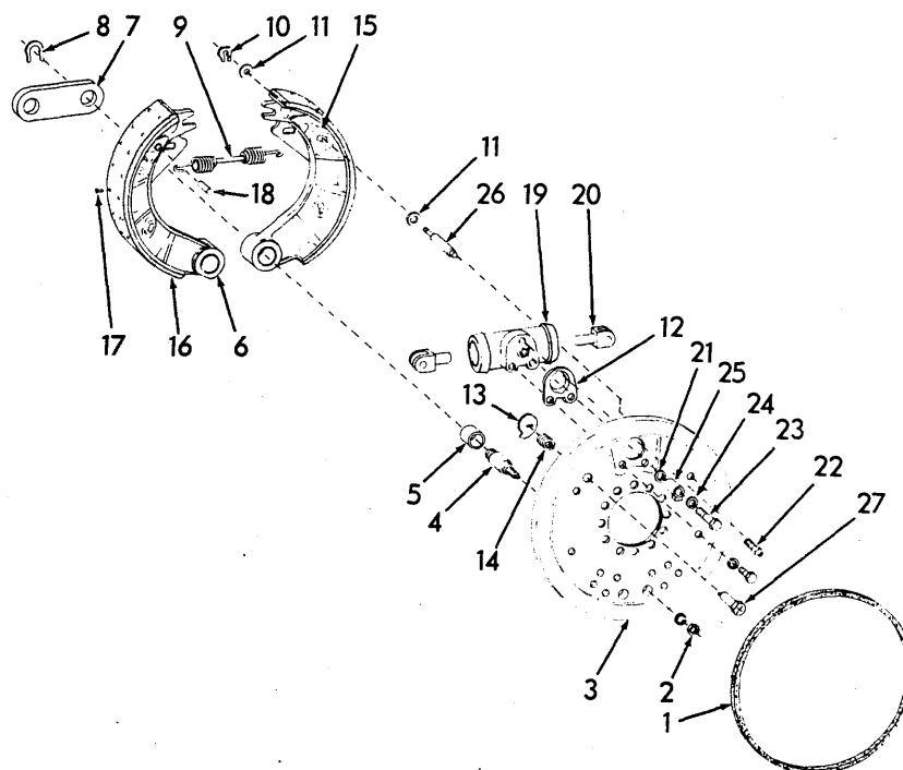
BR A K E A S S E M B L Y
